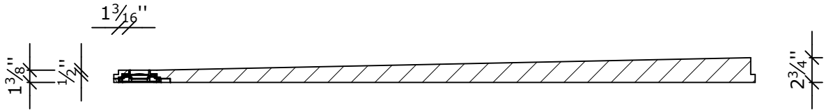
section A-A (1 : 15)
